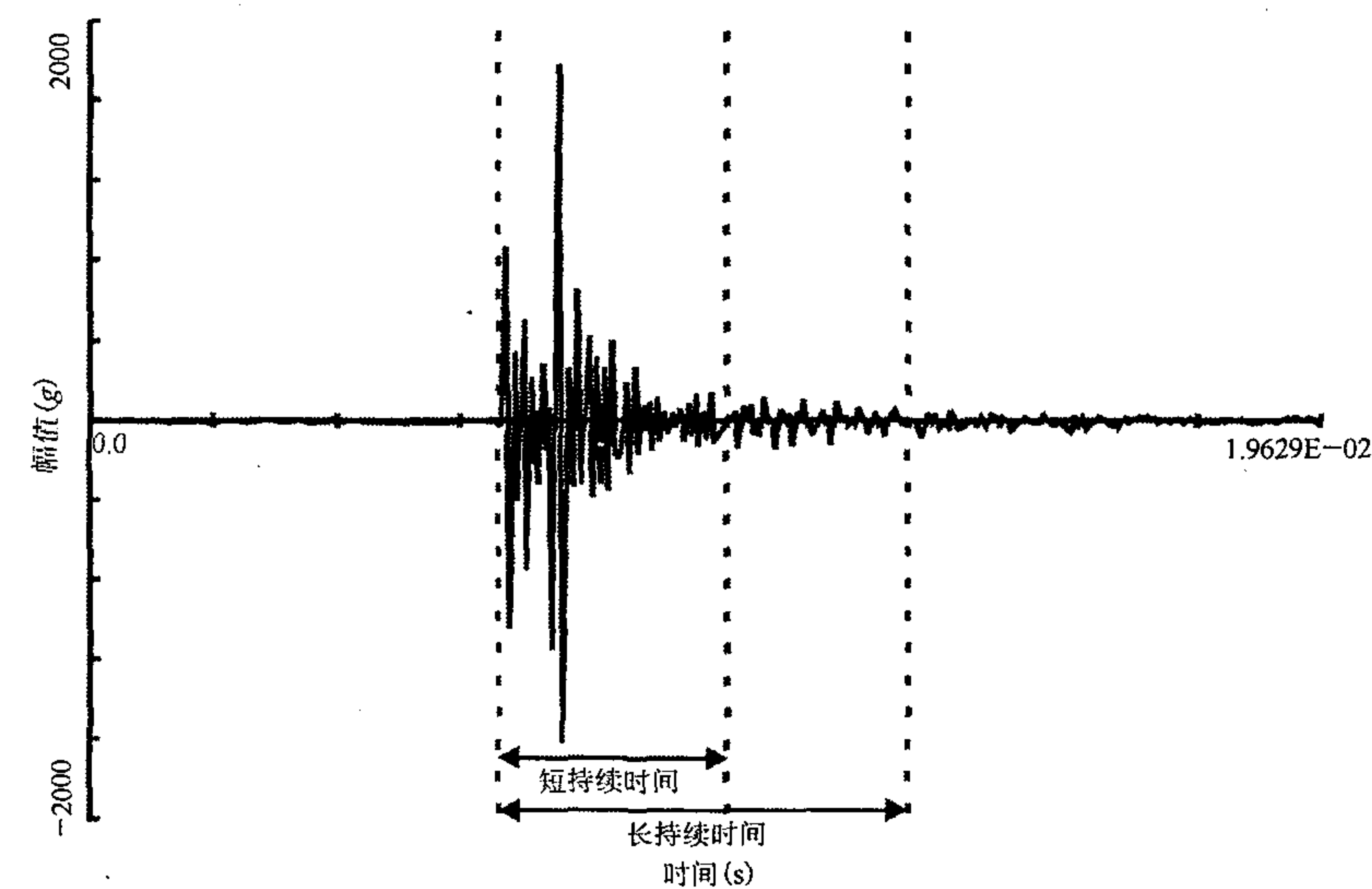
图 1 爆炸分离冲击的加速度时间历程
