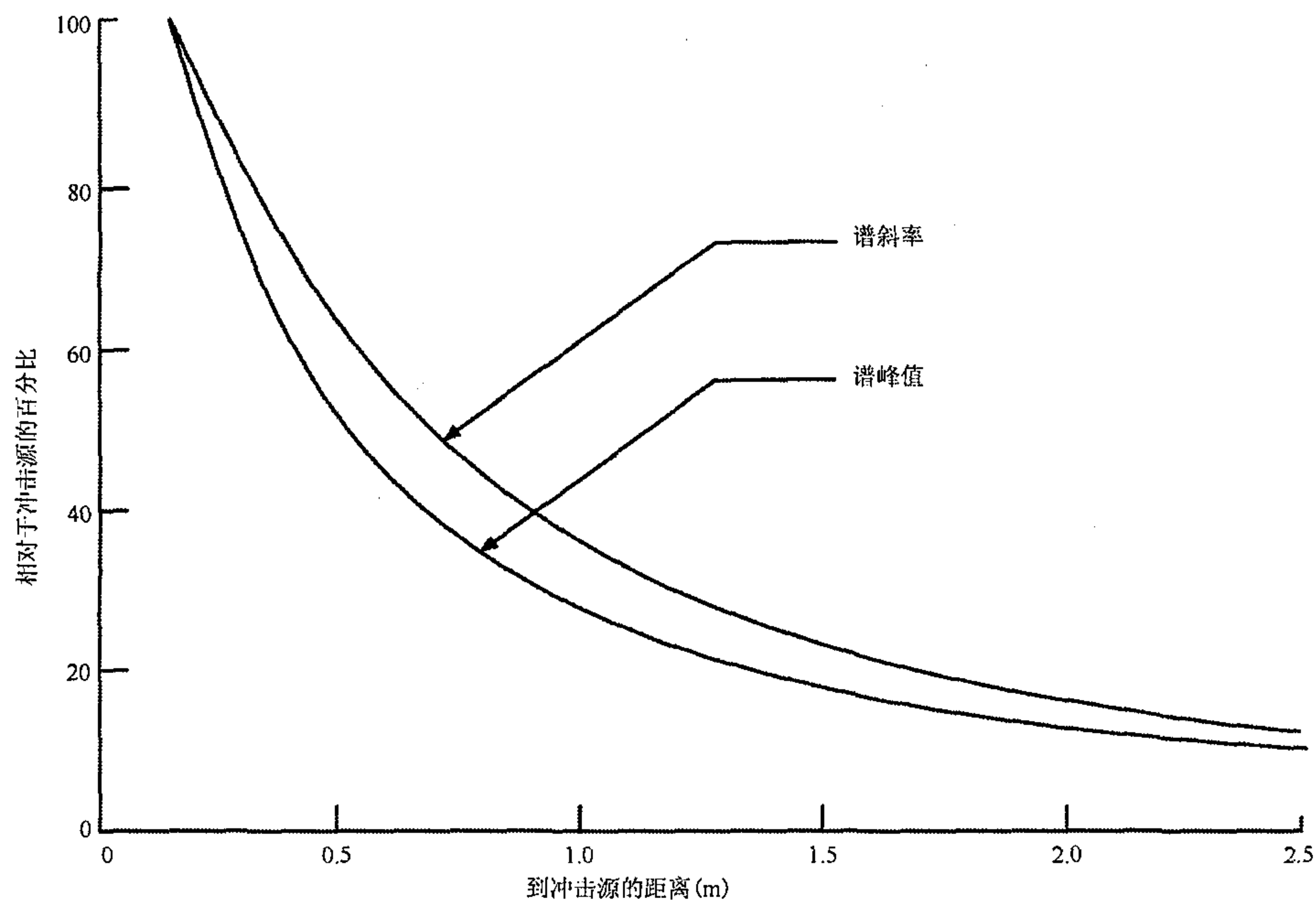
图 B. 2 冲击响应谱与到冲击源距离的关系
