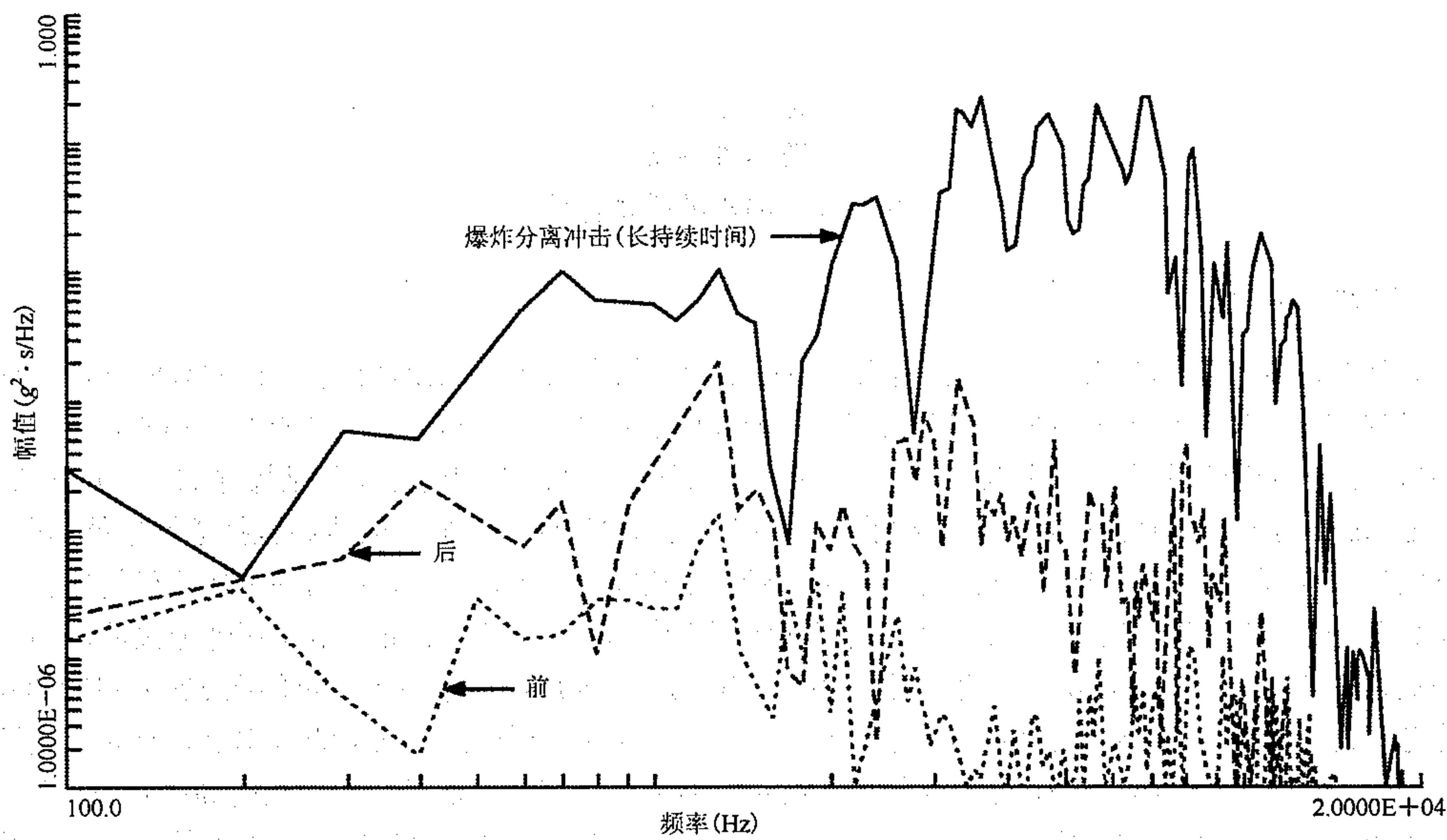
图 7 加速度能量谱密度估计
