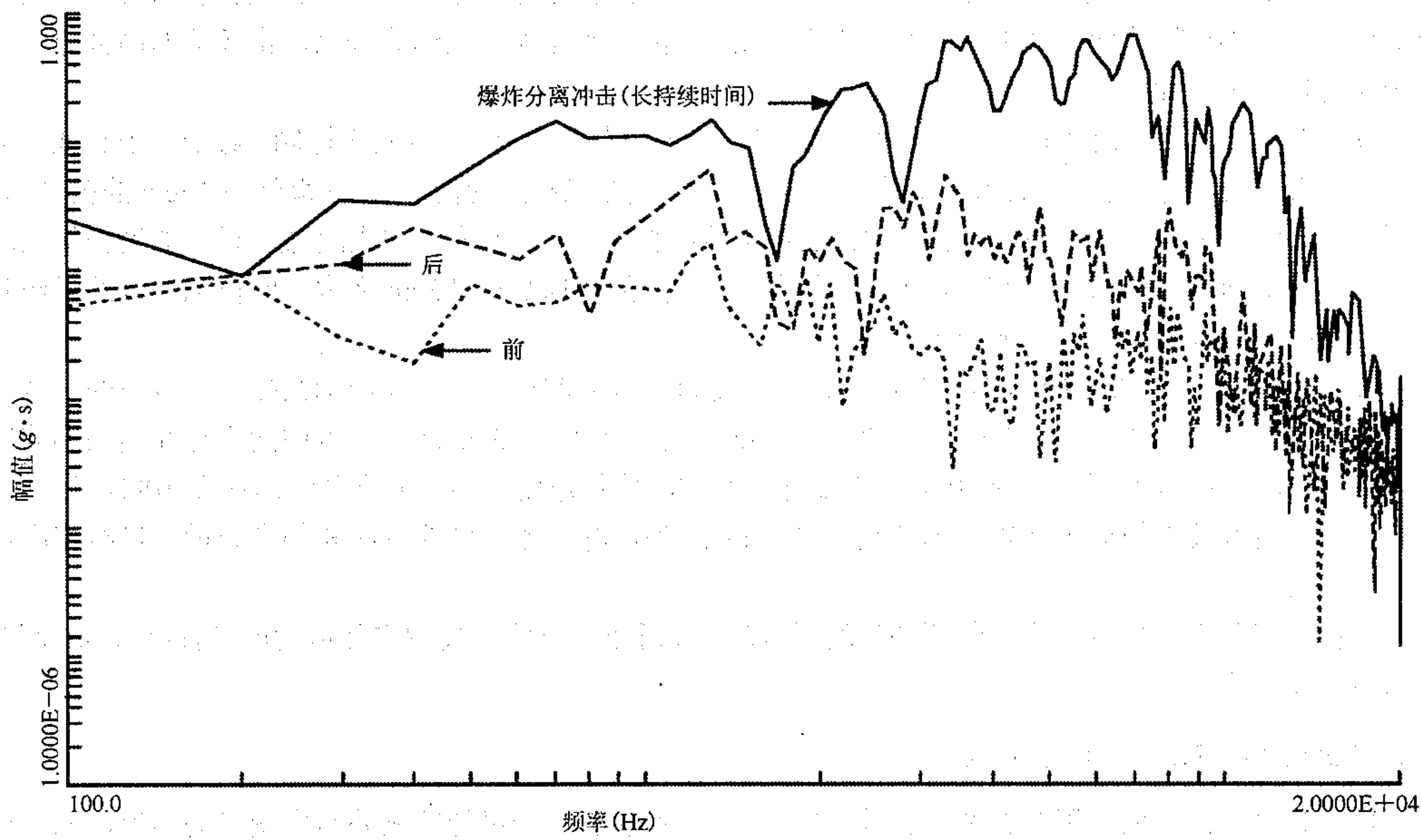
图 8 加速度傅立叶谱估计
