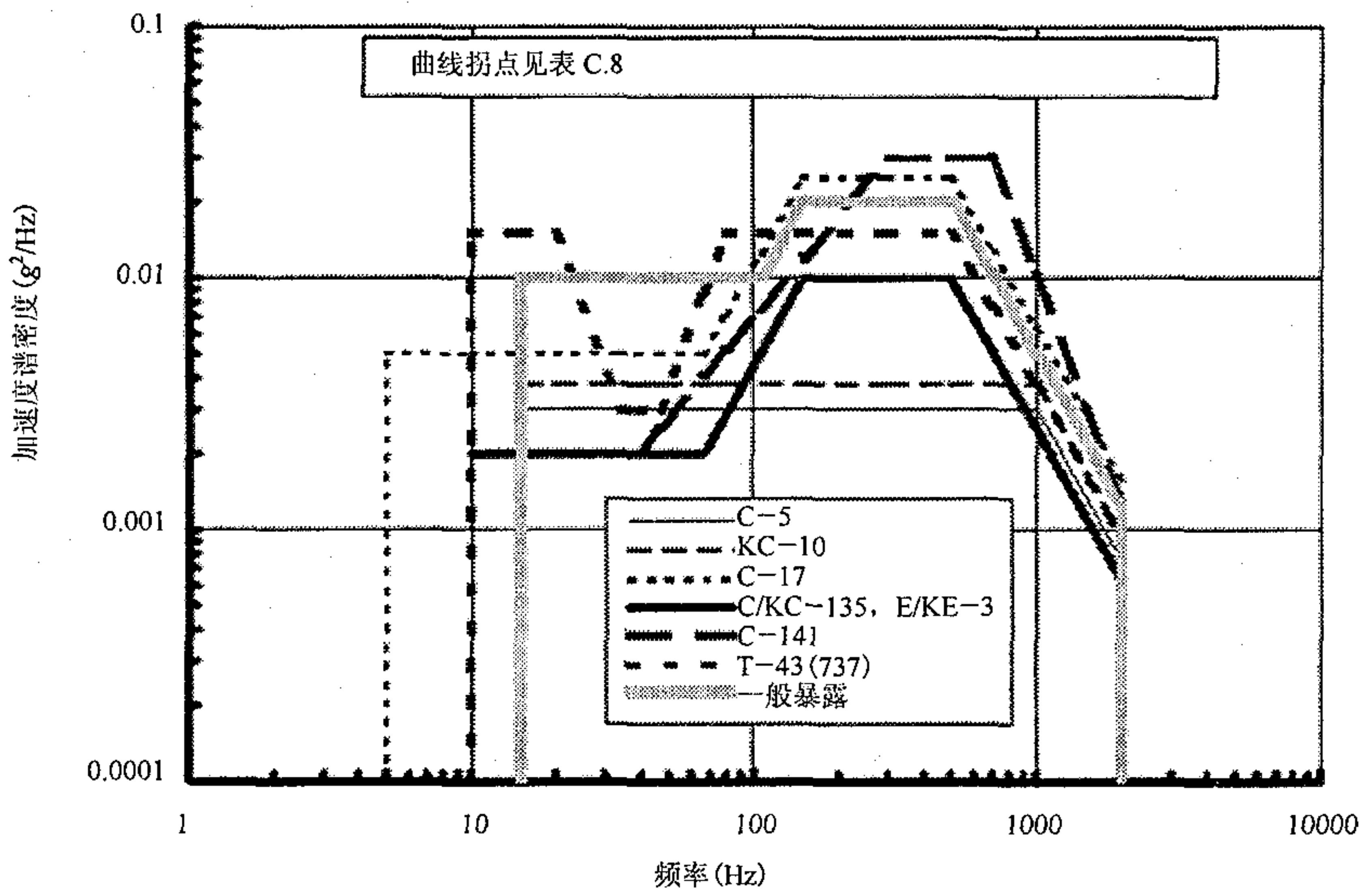
图 C. 6 喷气式飞机货物振动环境
